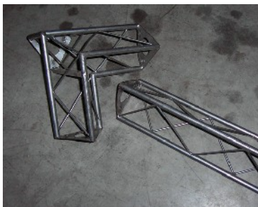
KIT STRUCTURE ACIER 150MM OPTIC PAR 575
