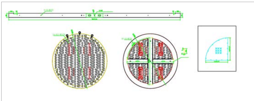
CERCLE VIDÉO LED D. 1100MM (AFFICHAGE 1000MM - RÉOLUTION : 500 X 500PX)
