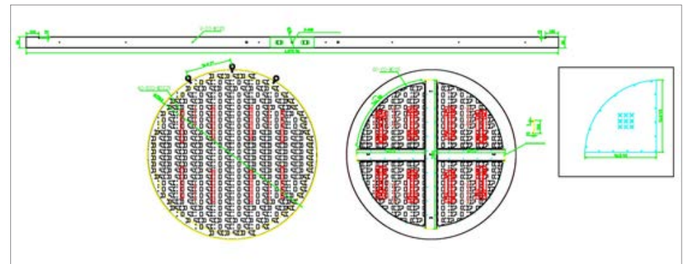
CERCLE VIDÉO LED D.1300MM (AFFICHAGE 1200MM - RÉOLUTION : 600 X 600PX)
