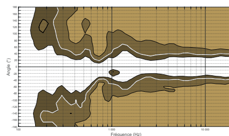
A15 Focus/Wide avec Panflex à 90° côté HF
