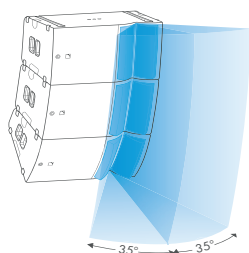
Panflex hybride à 70°/110°
